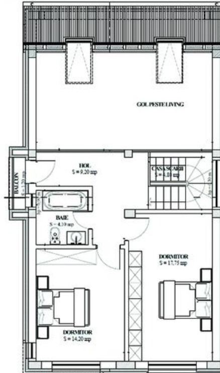
PLAN ETAJ
