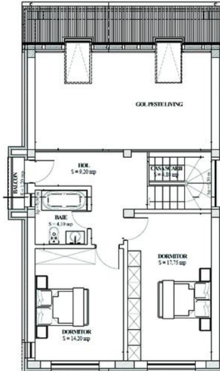
PLAN ETAJ
